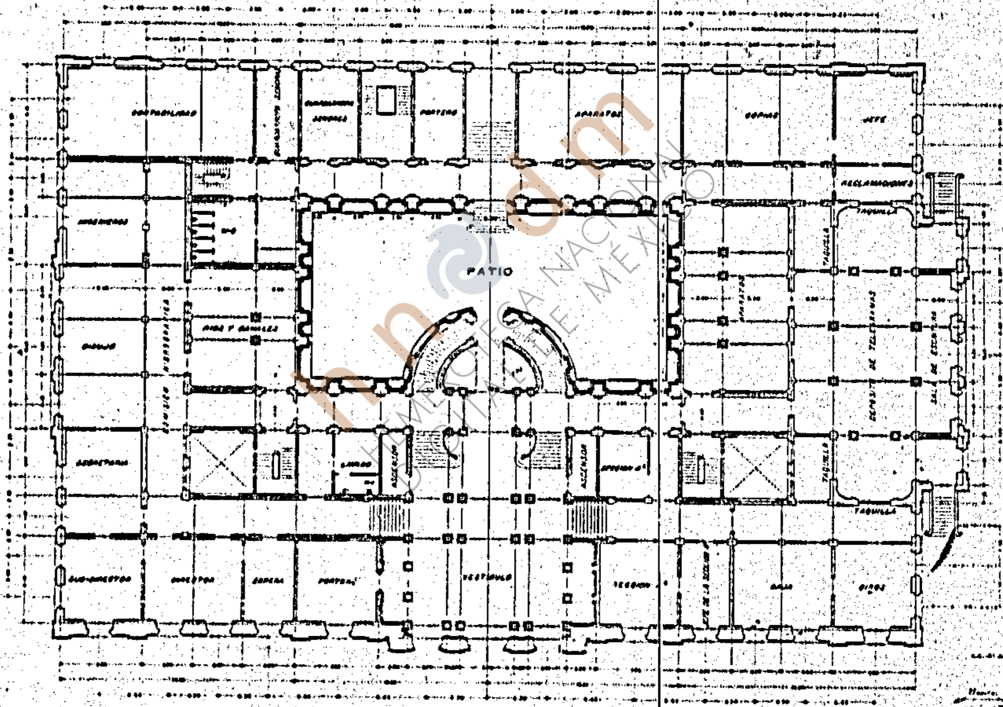
PLANTA DEL PISO BAJO.
