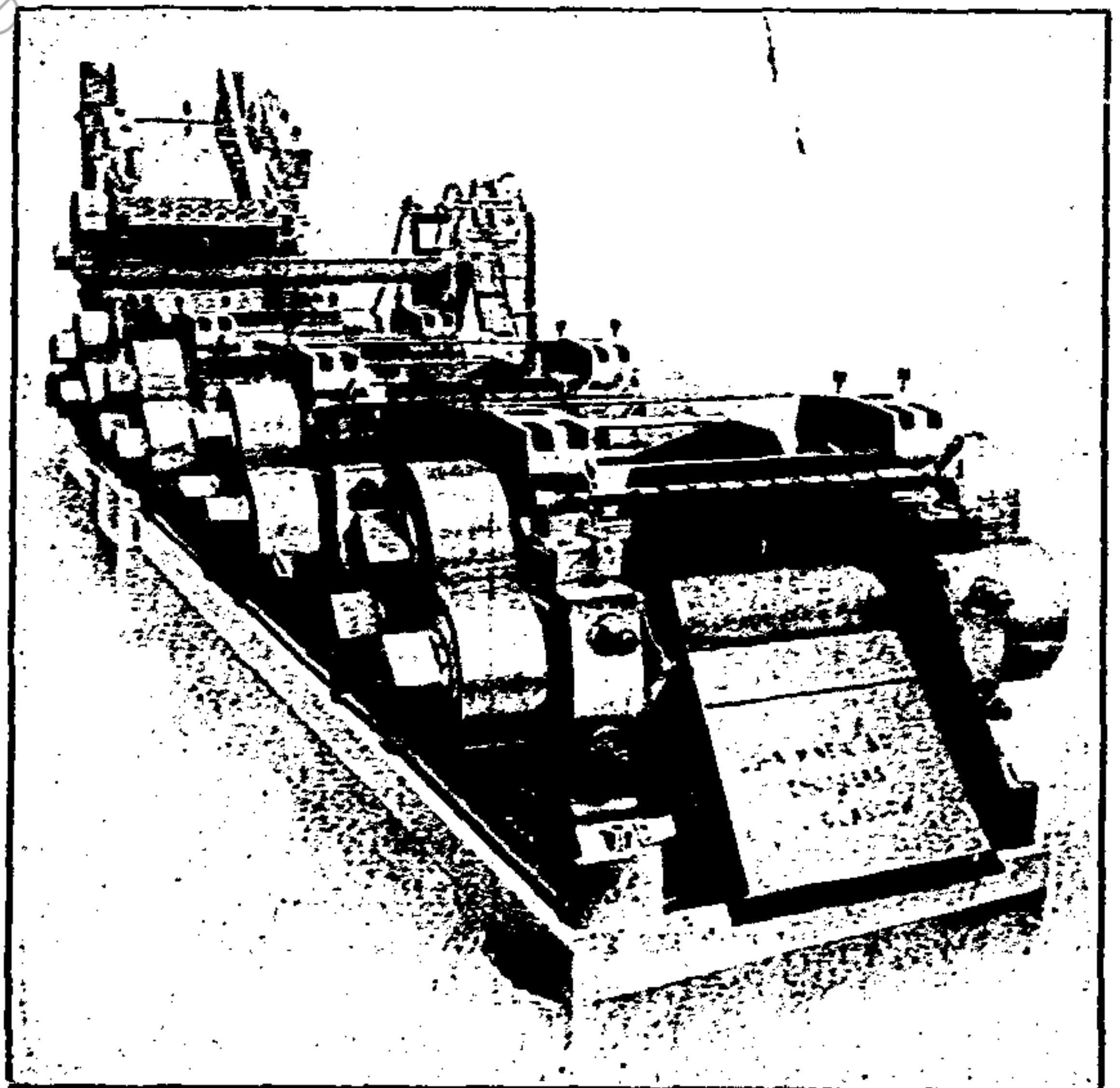
Trapiche del tipo "Dreadnought" de catorce moledores 34x75"
