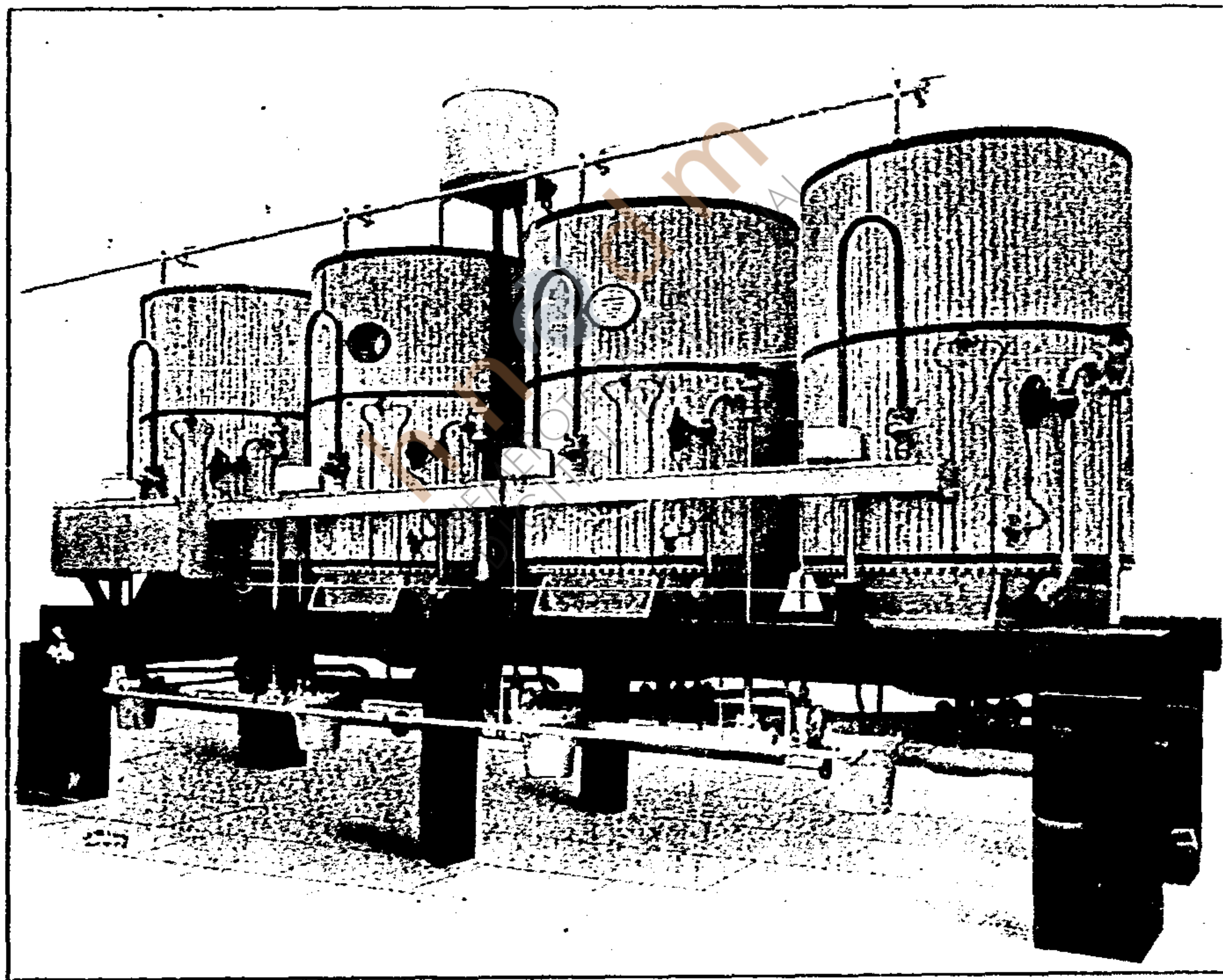
Una Bateria de las Defecadoras Continuas, Patente de Hatton, montada (en Plataforma temporaria) en los Talleres de los Sres. Fawcett Preston y Cia. Ltda., y embarcada recientemente para el extranjero
